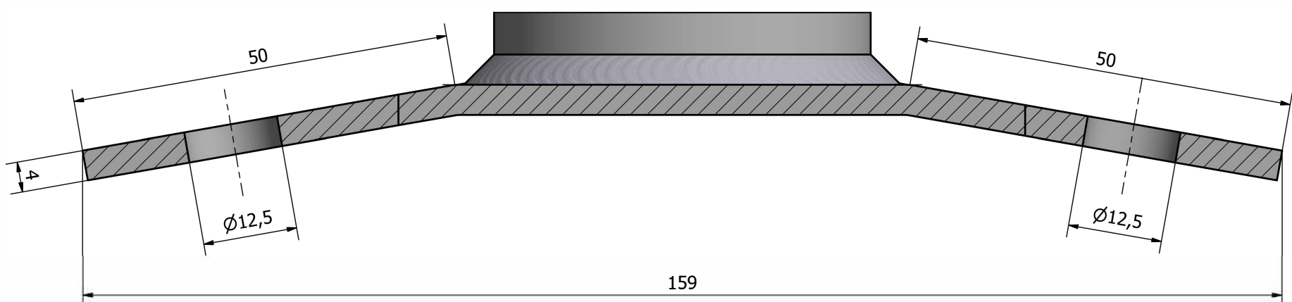
A-A ( 2:1 )
